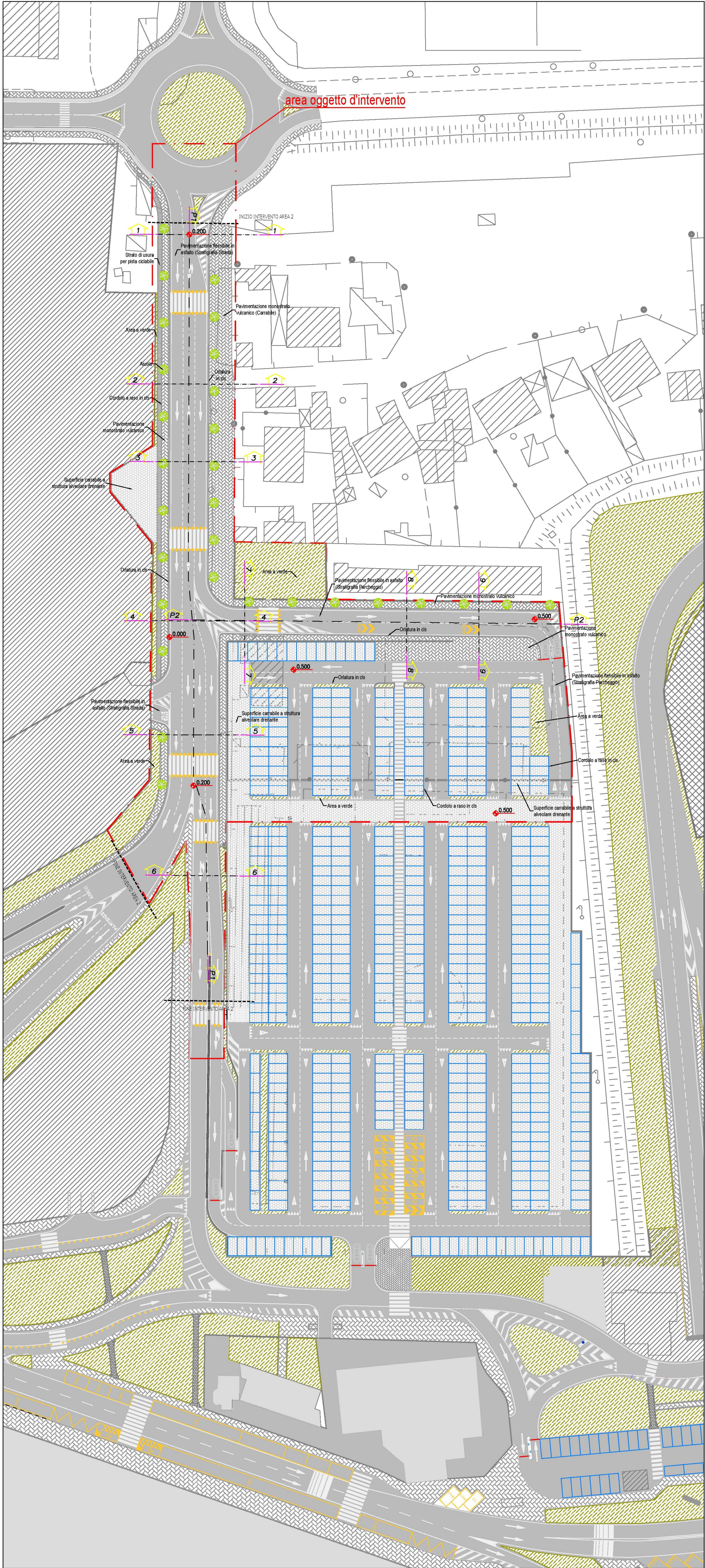
Planimetria di Progetto Scala 1:500
